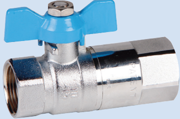
Art. 3123 Válvula esfera con retención Ball valve with check valve
